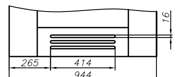
skrzydło SEMPRE „90” ze szczeliną wentylacyjną
