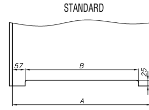
podcięcie wentylacyjne - dopłata 50 / 61,50
