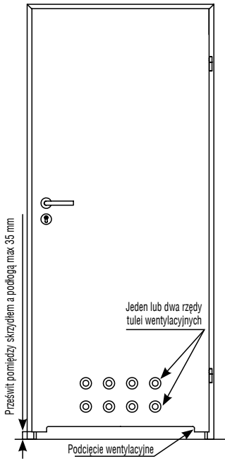
podcięcie wentylacyjne w skrzydłach bezprzylgowych z kolekcji FIESTA '09, NOBLE i DUO malowane - dopłata 50 / 61,50
