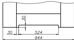
skrzydło SEMPRE „90” z podcięciem wentylacyjnym
