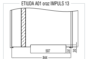
skrzydło Etiuda A01 „80” oraz Impuls 13 „80” z podcięciem wentylacyjnym – dopłata 50 / 61,50
