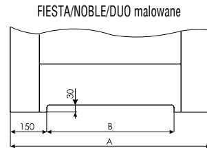
podcięcie wentylacyjne w skrzydłach bezprzylgowych z kolekcji FIESTA '09, NOBLE i DUO malowane - dopłata 50 / 61,50
