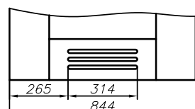
skrzydło SEMPRE „80” ze szczeliną wentylacyjną
