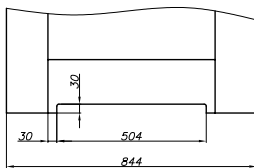
skrzydło ARCO „80” z podcięciem wentylacyjnym
