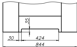
skrzydło SEMPRE „80” z podcięciem wentylacyjnym
