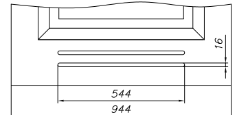
skrzydło VERTIGO „90” ze szczeliną wentylacyjną
