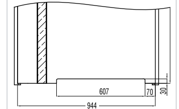
skrzydło Etiuda A01 „90” oraz Impuls 13 „90” z podcięciem wentylacyjnym – dopłata 50 / 61,50
