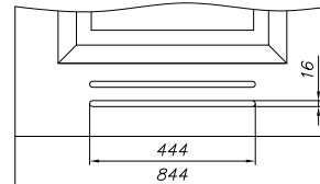
skrzydło VERTIGO „80” ze szczeliną wentylacyjną
