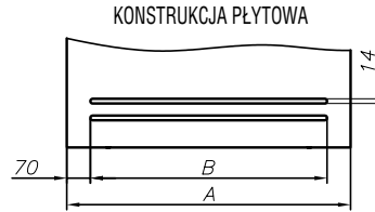
szczelina wentylacyjna w skrzydłach o konstrukcji płytowej – dopłata 70 / 86,10
