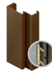
Ościeżnica metalowa kątowna
