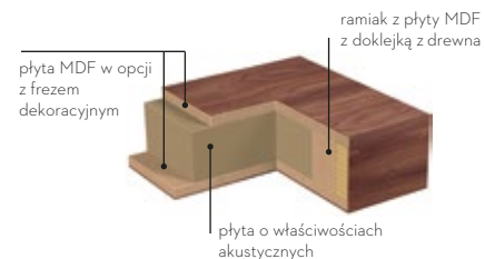
PRZEKRÓJ SKRZYDŁA ANDORA, BOLZANO
