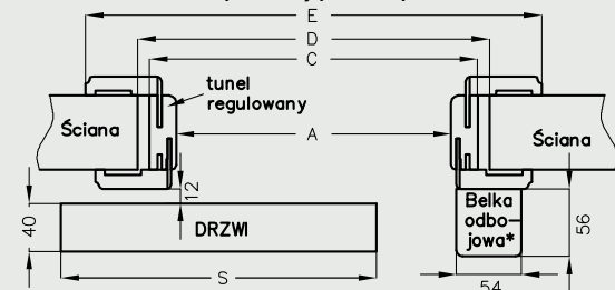
NT - przekrój poziomy
