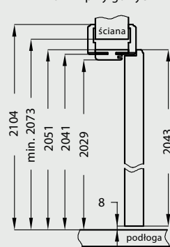
wymagana wysokość otworu w murze 2073 mm
