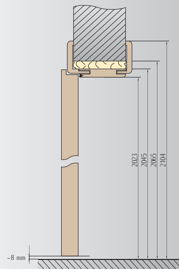
Zakres regulacji ościeżnicy regulowanej
