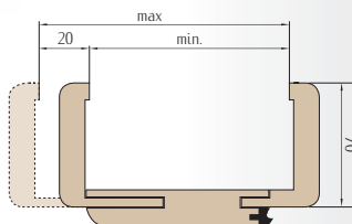
Zakres regulacji ościeżnicy regulowanej
