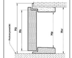
Rysunek poglądowy dla ościeżnicy i progów dla: FTP SL
