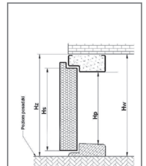
Rysunek poglądowy dla ościeżnic i progów dla: FAP SL, FRP SL, ALUTERM, FA SL z przekładką.
