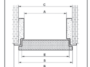
Rysunek poglądowy dla ościeżnicy: FTP SL
