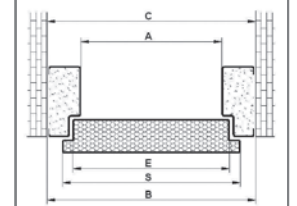
Rysunek poglądowy dla ościeżnic: FAP SL, FRP SL, ALUTERM, FA SL z przekładką
