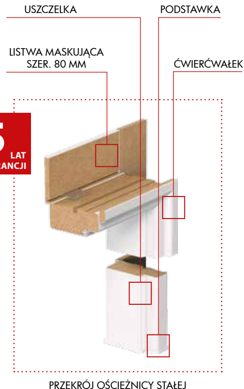
PRZEKRÓJ OŚCIEŻNICY STAŁEJ
