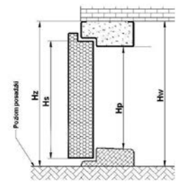
Rysunek poglądowy dla ościeżnic drzwi i progów dla: FD, FC, FR, FR SL, FA SL, FA SL PREMIUM, FR SL PREMIUM, FR PREMIUM, FC PREMIUM
