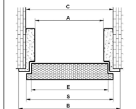
Rysunek poglądowy dla ościeżnic FN, FT PREMIUM, FT SL, FT SL PREMIUM
