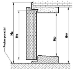
Rysunek poglądowy dla ościeżnic drzwi i progów dla: FN, FT SL, FT PREMIUM, FT SL PREMIUM
