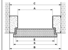
Rysunek poglądowy dla ościeżnic FC, FD, FR, FR SL, FA SL, FA SL PREMIUM, FR SL PREMIUM, FR PREMIUM, FC PREMIUM
