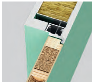
Przeciwpzylga (otwierane do wewnątrz) - drzwi lewe
