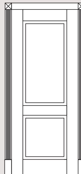
OPASKI OZDOBNE OP-4 KOPERTY GÓRNE SŁUPKI DOLNE (PRZYKŁAD MODEL PP-0) Opcja za dopłatą
