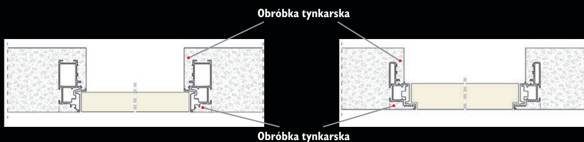
Ościeznica ukryta standard
