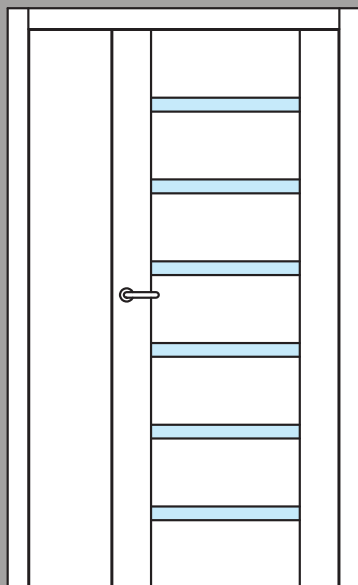
Przykładowe drzwi dwuskrzydłowe asymetryczne z dostawką pełną (model WE-6)
